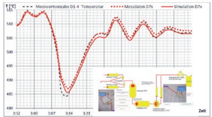
Dynamische Simulation einer Frischdampfleitung
