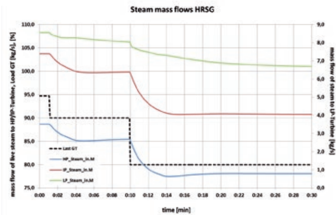
Zeitentwicklung der Dampfströme vom Abhitzekegel einer GUD-Anlage
